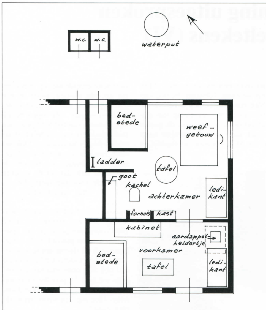
Plattegrond van de weverswoning van Jaonneke Janssens, Hasseltstraat 231, Tilburg (ca. 1900). Reconstructie Ton Wagemakers (tekening John Goeijers, gemeente-archief 1985)
